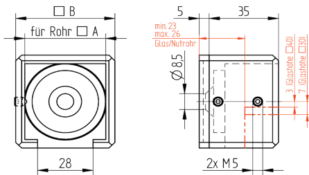
Abbildung Variante rechts
